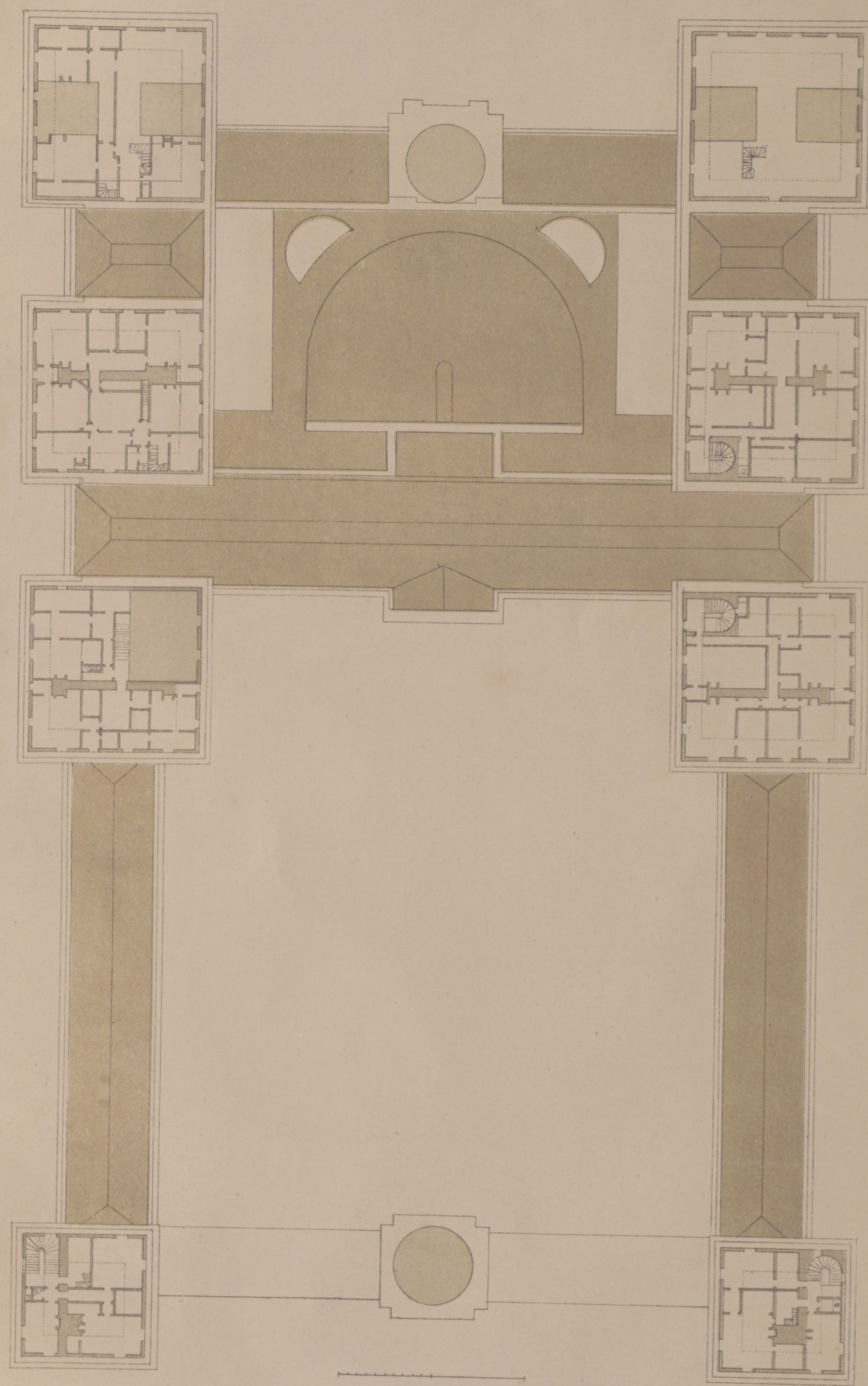
PLAN DE L'ÉTAGE EN MANSARDES
